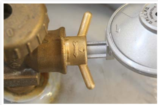
Vänstergängad anslutning
